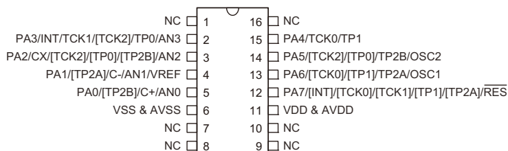
HT66F04 16 NSOP-A
