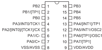
HT68F016 16 DIP-A/NSOP-A/SSOP-A
