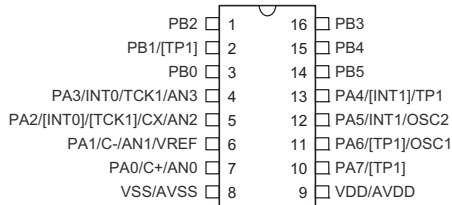
HT66F016 16 DIP-A/NSOP-A/SSOP-A
